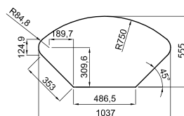
Wymiary wycięcia (mm)
