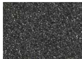
hedenbergit 9011
