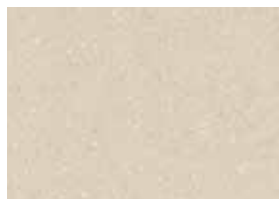
cryolite 5196
