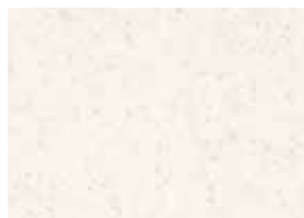
wollastonite 1076
